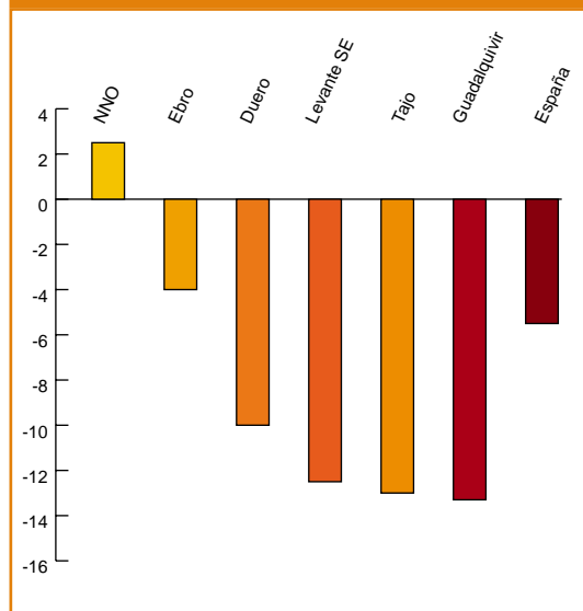
Figura 4. Tendencia de la precipitación en cuencas españolas (1947-1999)
