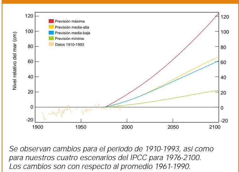
Figura 2. Cambios en el nivel del mar en lagos (37.1°N 8.67W) en el extremo sur de Portugal (150 km al oeste del Parque Nacional de Doñana)
