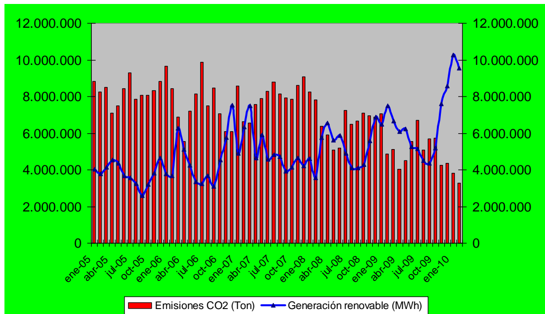
Evolución mensual de las emisiones de CO 2 y la generación con energías renovables del sistema eléctrico peninsular (Enero 2005-Febrero 2010).
